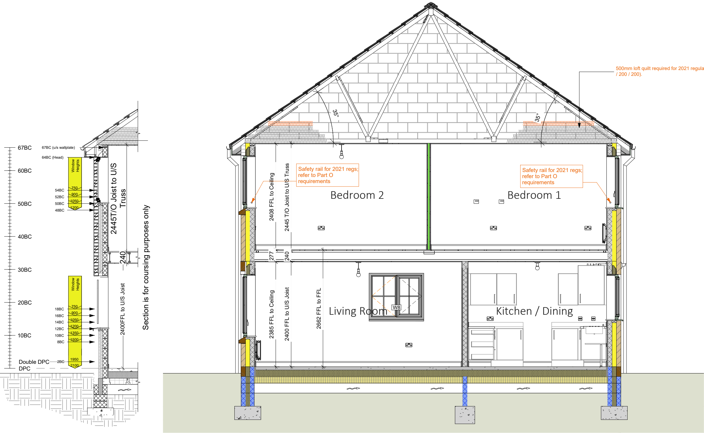
A Section A - A 1 : 50
